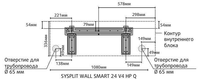
Табл. 2. Габариты внутреннего блока
